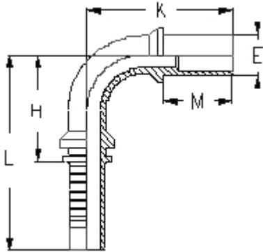
Фитинг 90° BEL (под врезное кольцо и гайку, для соединения рукава с трубой)
