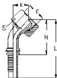
Фитинг DKL (гайка) 45° (внутренняя метрическая резьба, наружный универсальный конус 24°/60°)
