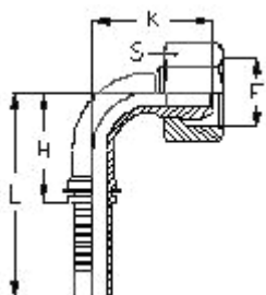
Фитинг DKL (гайка) 90° (внутренняя метрическая резьба, наружный универсальный конус 24°/60°)
