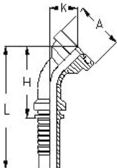
Фитинг 45° SFL (фланец) (легкая серия)
